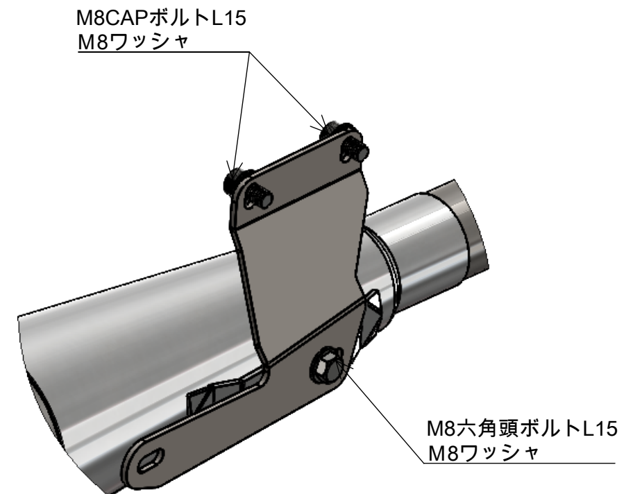
詳細図 A スケール 2 : 5
