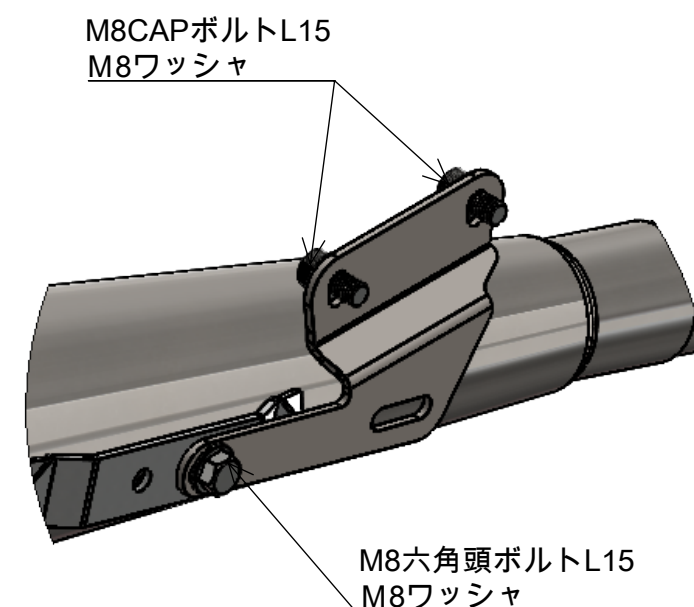
詳細図 A スケール 2 : 5
