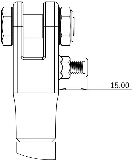
詳細図 A
