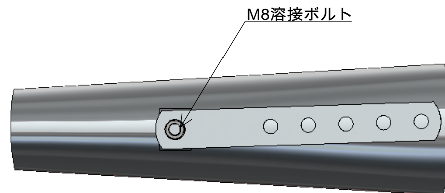
詳細図 A スケール 2:5
