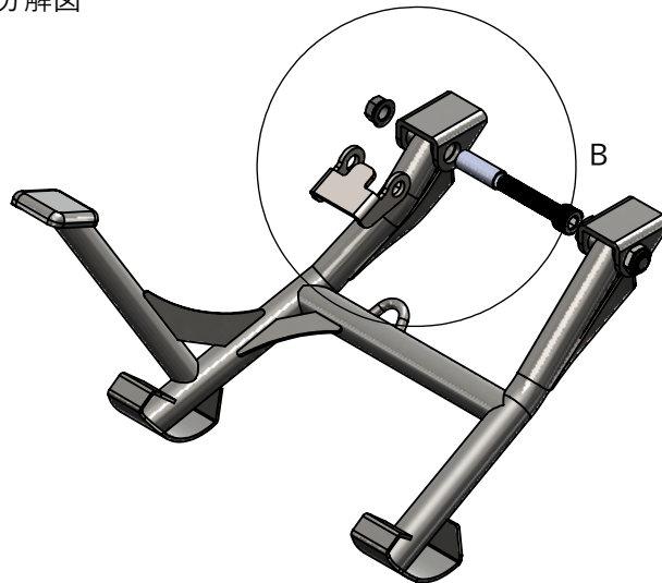
分解図
